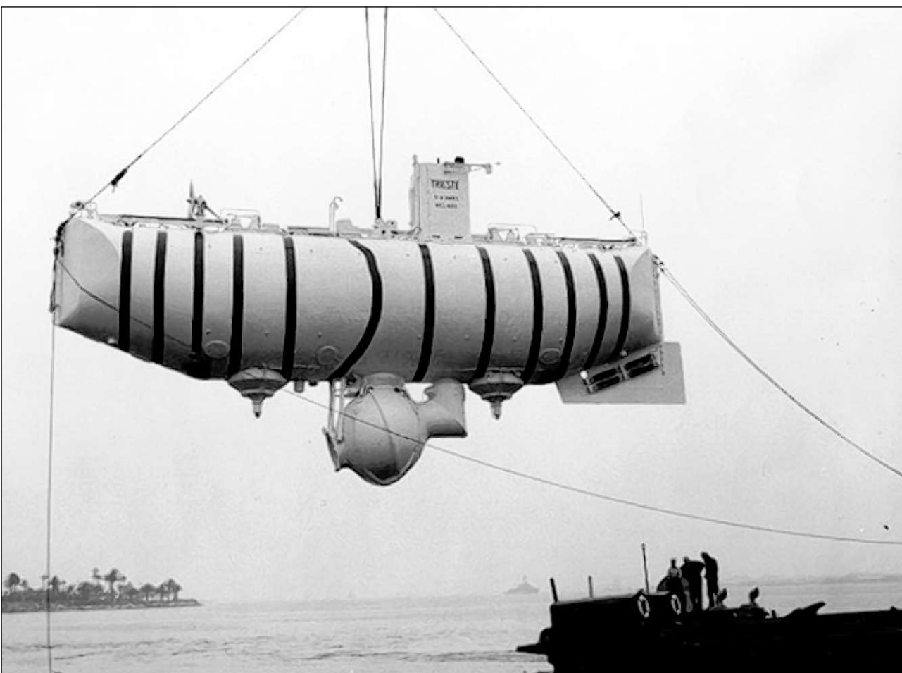
Il sutmarin «Trieste» sviluppa dad Auguste e Jacques Piccard. (Fotografia dal 1958).
