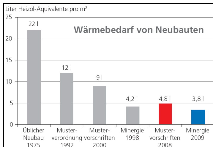
Illustraziun 3: Basegn da chalur d'edifizis novs en liters equivalents d'ieli da stgandar per m 2 surfatscha d'auzadas
