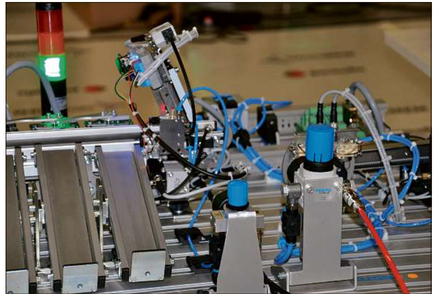
Il model per zavarar tocca han ils dus automaticchers sursilvans stui bajegiari e programmar entaifer mo in di.
